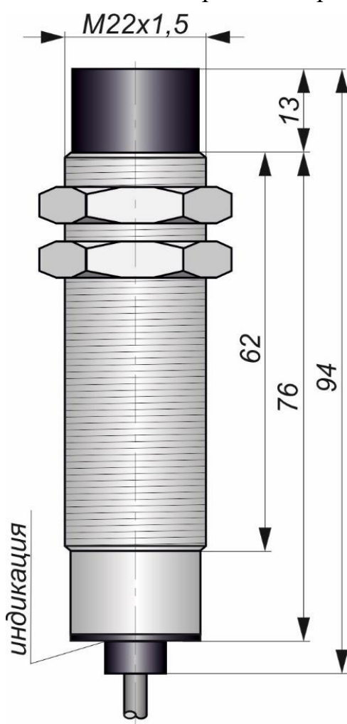
Габаритный чертеж
